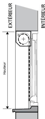
POSE EN TABLEAU ENROULEMENT EXTÉRIEUR
