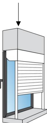
Hauteur réduite par le caisson et porte visible de l'extérieure
