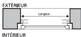
POSE EN TABLEAU ENROULEMENT EXTÉRIEUR
